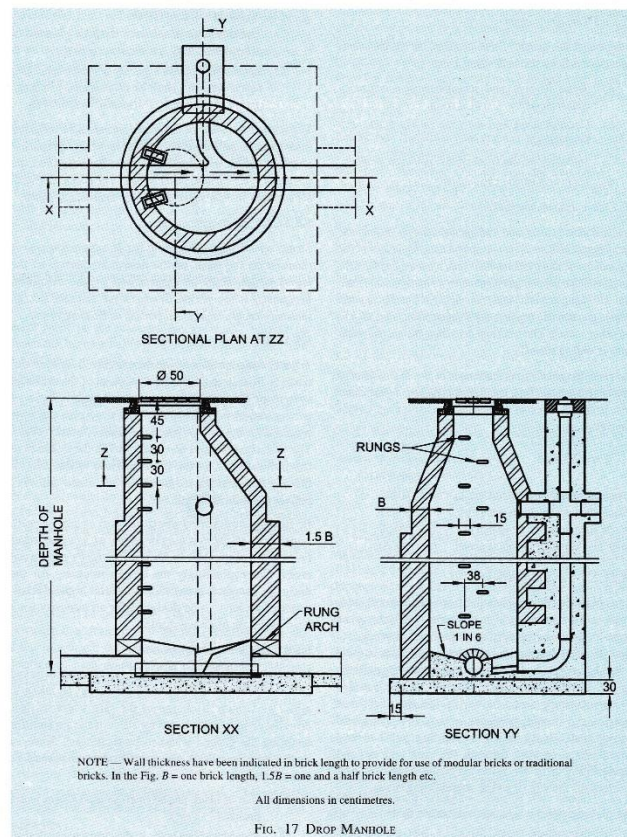
FIG. 17 DROP MANHOLE
